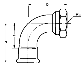
メスアダプタ付90°エルボ
