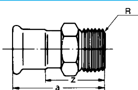
オスアダプタ付ソケット1型
