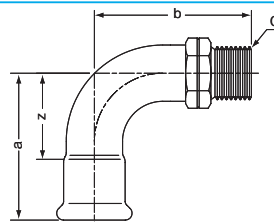
オスアダプタ付90°エルボJ型
