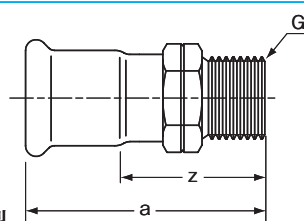
オスアダプタ付ソケットJ型
