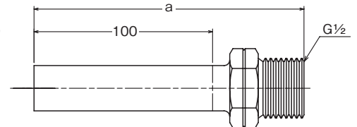
オスアダプタ付短管J型
