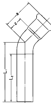
片ソケット45°エルボ
