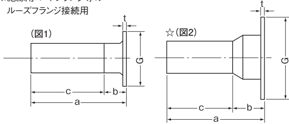
ラップ付短管
