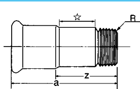
オスアダプタ付ソケット2型
