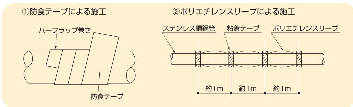
図3-1-1 防食方法
