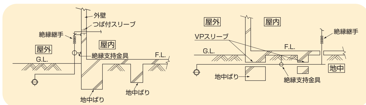
図3-1-2 絶縁継手の施工例（参考）
