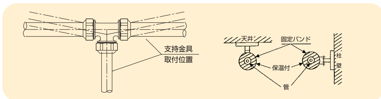
図8-5-1 支持金物の取り付け位置 図8-5-2 熱膨張による伸縮が大きい配管の支持方法
