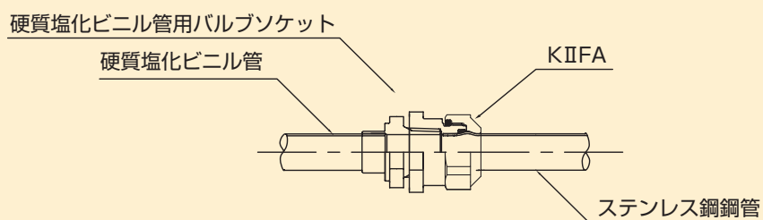
図2-10-5 硬質塩化ビニル管とのねじ接合
