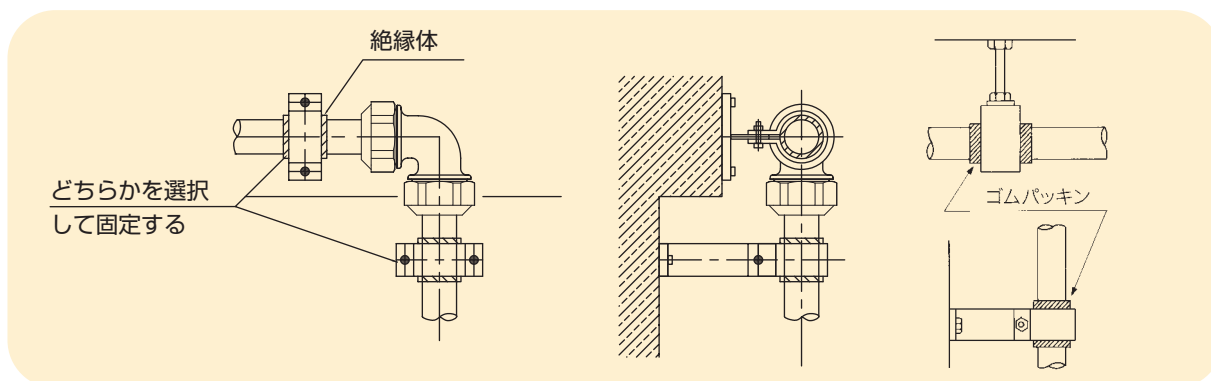
図8-4 絶縁材を使用して支持
