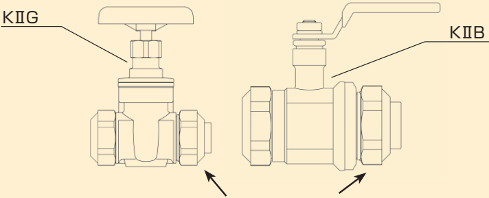
水圧テストプラグ（KⅡTPLG）で閉止する（13Suは袋ナットとキャップを使用）
