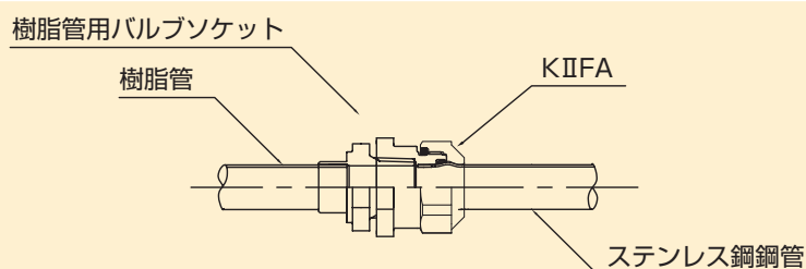
図2-10-6 樹脂管とのねじ接合
