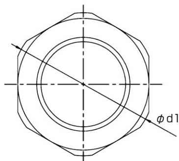
BKジョイントⅡ袋ナット外径寸法
