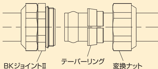
BKジョイントⅡと変換ナットの接合
