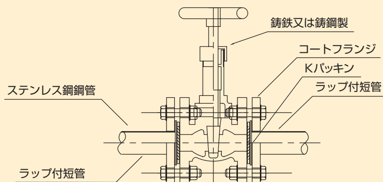
図2-12 バルブとのフランジ接合
