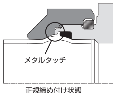
正規締め付け状態
