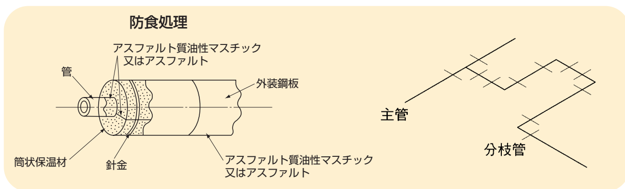
図3-2 防食処理
