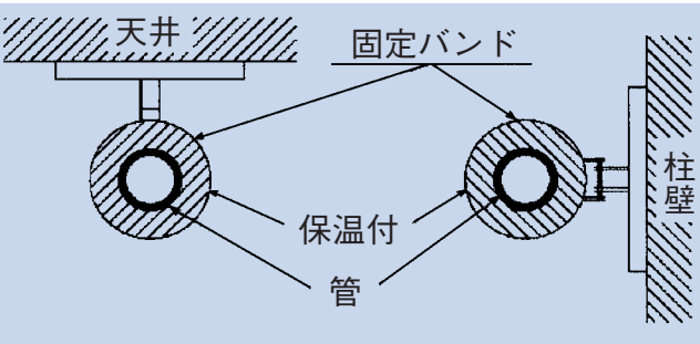
図9-5-2 熱膨張による伸縮が大きい配管の支持方法
