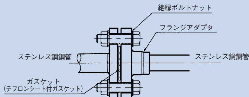
図3-6 電気機器との接合
