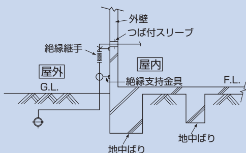
図4-1-2 絶縁継手の施工例（参考）
