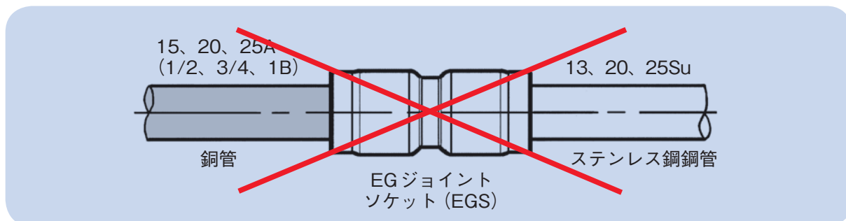
図3－5－4 銅管との直接接合は不可
