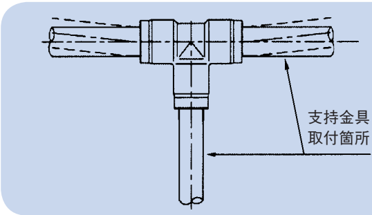
図9-5-1 支持金物の取り付け位置
