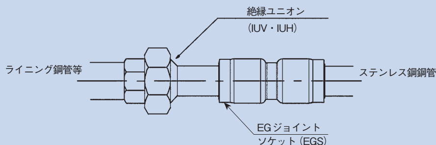
図3－5－2 絶縁ユニオンによる接合
