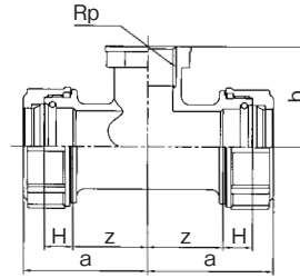
水栓ティー
